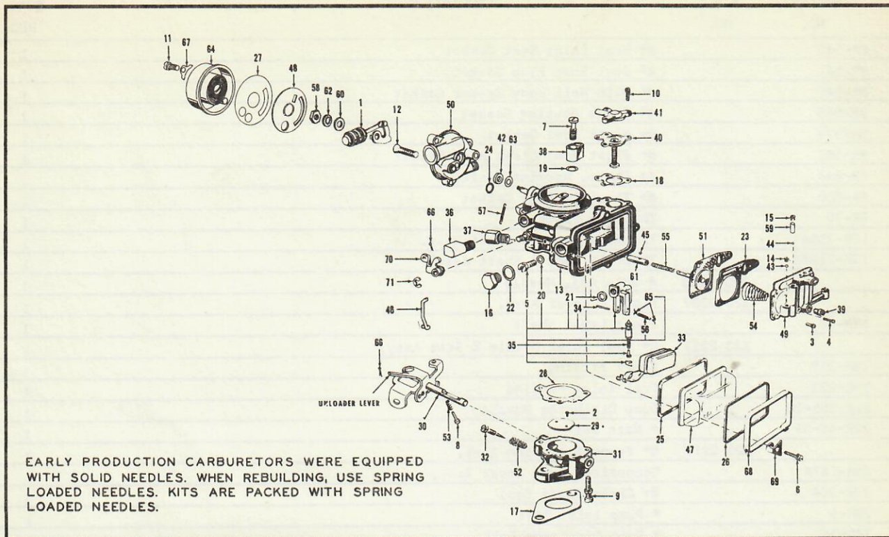
CARBURETOR 59 10 (LDT)
